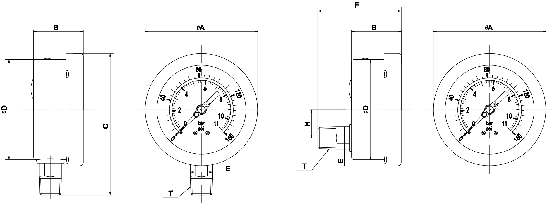
100外卡压力表
